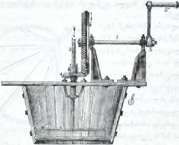
სურ. 17.—ბაბოს ჩასაბერავი მანქანა.
