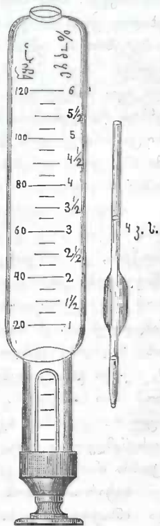
სურათი 10. ფეგელის ლაქტოსკოპი თავის პიპეტით.
