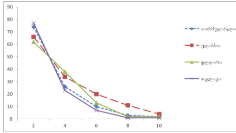
ნახ. 3.4.1. ქარის აქტიური და არააქტიური სიჩქარეების V(m/v) , განმეორადობა (P%) წელიწადში.
