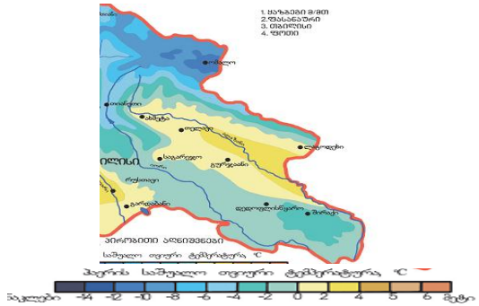
ნახ. 2.1.3. ჰაერის ტემპერატურა (იანვარი)
