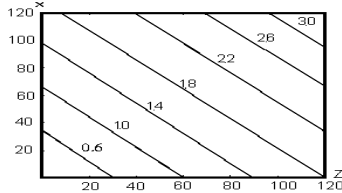
ნახ. 4.4.2 სიმინდის კულტურის მოსავლის (ტ/ჰა) დამოკიდებულება ატმოსფერულ ნალექებზე-x (მმ) და ნიადაგის (20სმ სიღრმეში) პროდუქტიულ ტენზე-z (მმ), VI-VII თვეებში
