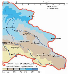
ნახ. 2.2.2. ჰაერის შეფარდებითი სინოტივე (%). ივლისი
