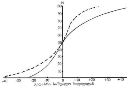
ნახ. 4.3.1 ბოლო (-) და პირველი (----) წაყინვების აღბათობის მრუდები (%)
